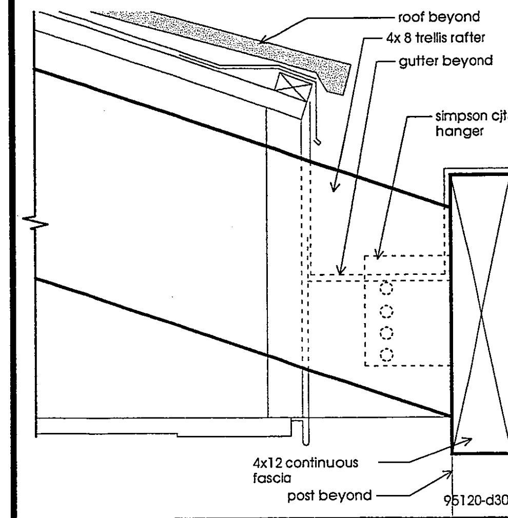
FASCIA AT TRELLIS Scale: 3" = 1'-0" 8
